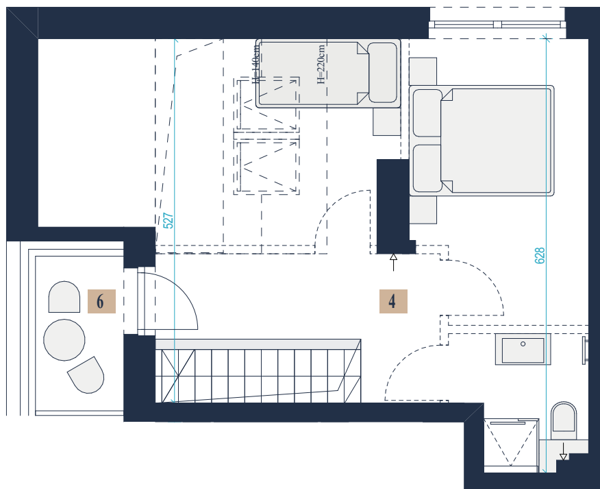
POZIOM 2
