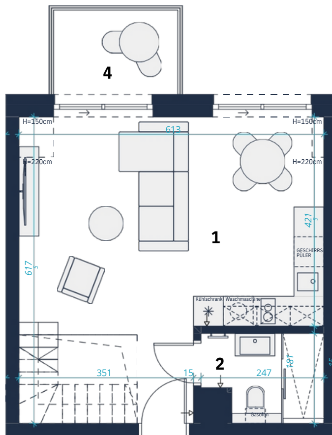
Untergeschoss
