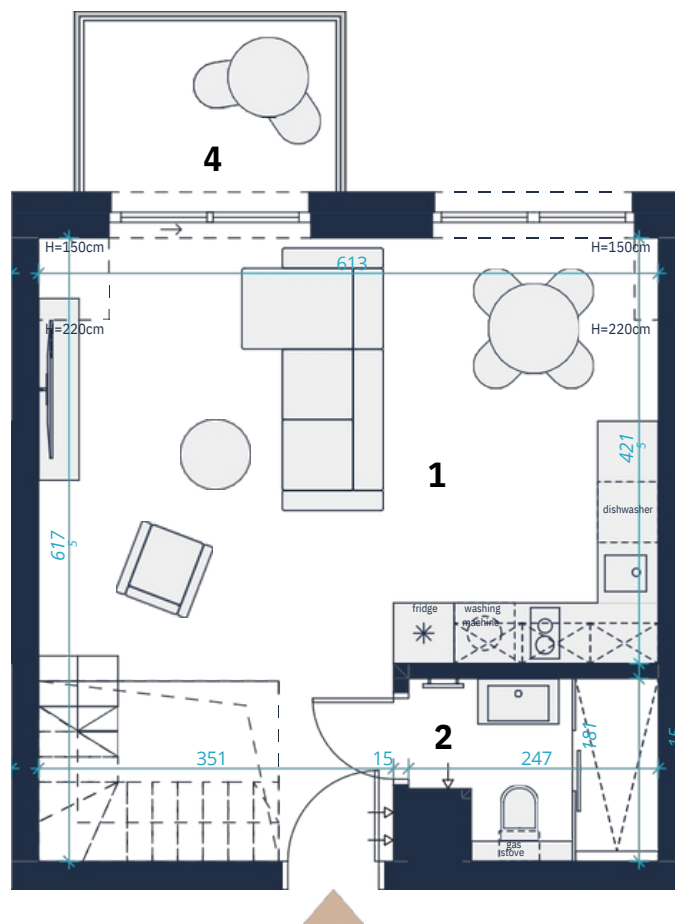
První nadzemní podlaží
