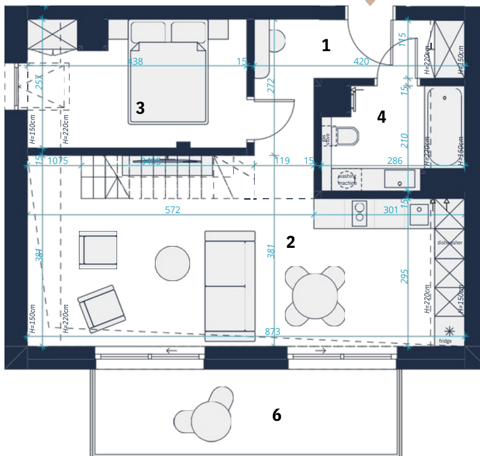
První nadzemní podlaží
